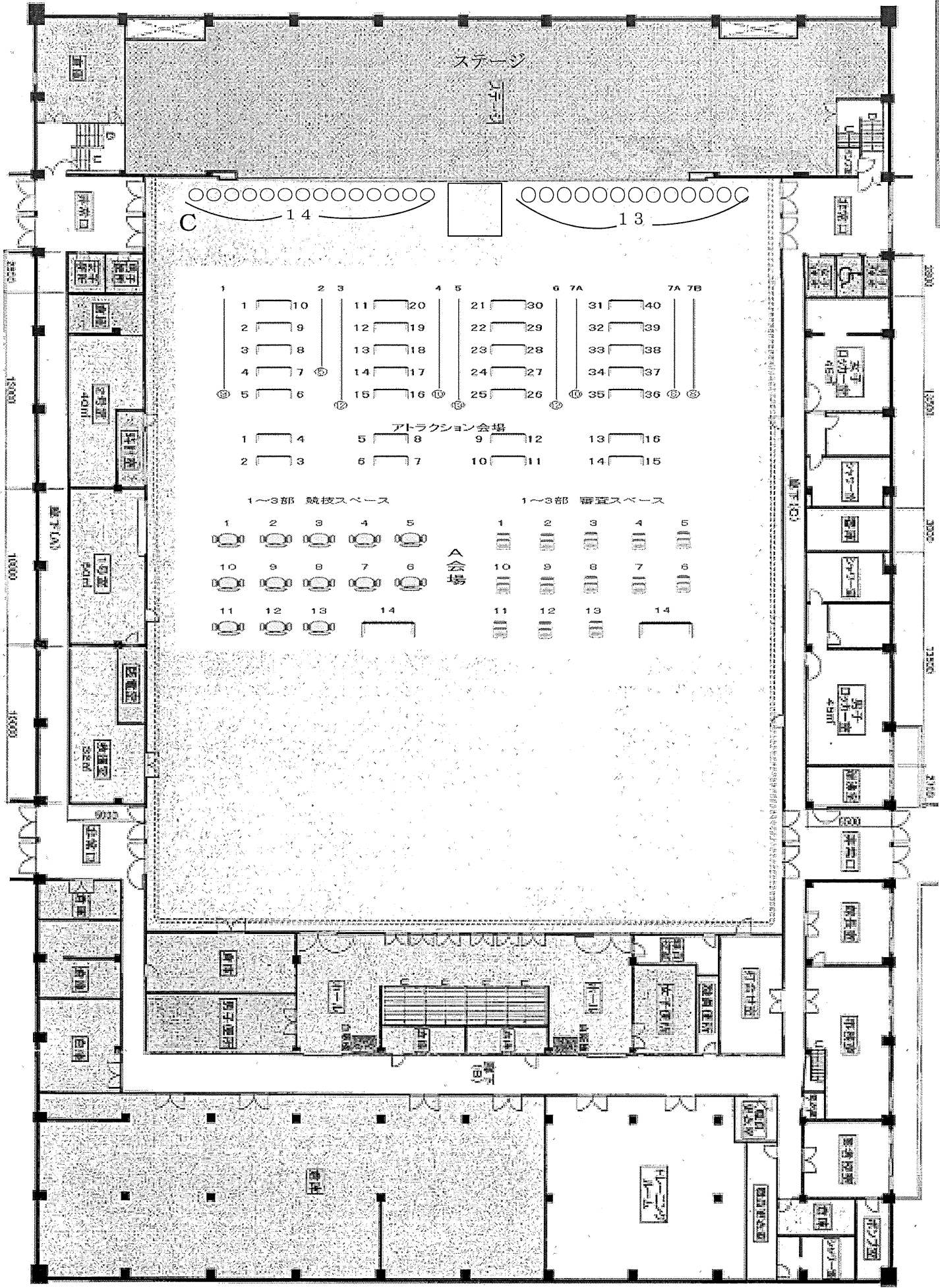
横浜文化体育館階平面図
